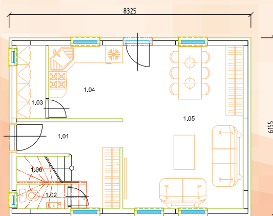
prízemie
