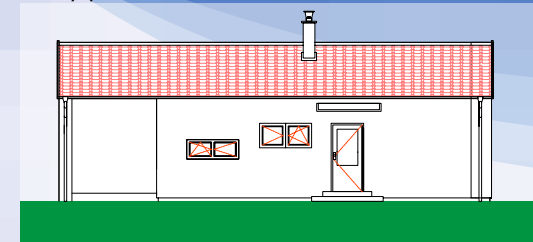
zadný pohľad
